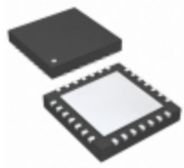
PIC18LF2423T-I/ML Microchip Technology IC MCU 8BIT 16KB FLASH 28QFN
