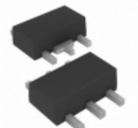
RT9069-C0GX5 Richtek USA Inc. IC REG LDO 12V 0.2A SOT89-5
