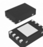
ISL8009AIRZ-T7A Intersil IC REG BUCK ADJ 1.5A SYNC 8DFN
