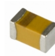
TLCL476M002RTA AVX Corporation CAP TANT 47UF 2V 20% 0603
