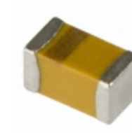
TLCL476M004RTA AVX Corporation CAP TANT 47UF 4V 20% 0603
