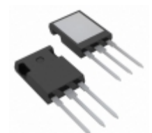
IXFR21N100Q IXYS MOSFET N-CH 1KV 18A ISOPLUS247
