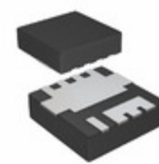
C3D1P7060Q Cree Wolfspeed DIODE SCHOTTKY 600V 1.7A 10PQFN
