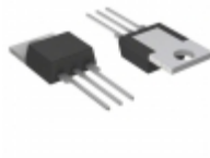
L2008L8 Littelfuse Inc. TRIAC SENS GATE 200V 8A TO220
