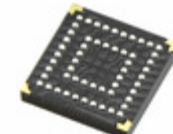
XCR3064XL-6CP56C Xilinx Inc. IC CPLD 64MC 5.5NS 56CSP
