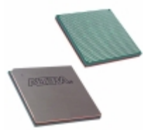
EP1SGX25FF1020C6 Altera IC FPGA 607 I/O 1020FBGA
