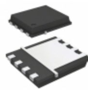
BSZ086P03NS3GATMA1 International Rectifier (Infineon Technologies) MOSFET P-CH 30V 40A TSDSON-8
