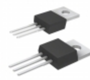
IXGP24N60C4D1 IXYS IGBT 600V 56A 190W TO220
