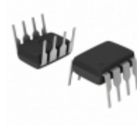
IXDD414PI IXYS IC MOSFET DRIVER LS 14A SGL 8DIP
