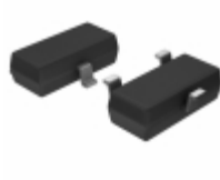
MMBZ5252C-HE3-08 Electro-Films (EFI) / Vishay DIODE ZENER 24V 225MW SOT23-3
