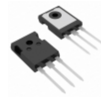
IXGH10N170 IXYS IGBT 1700V 20A 110W TO247
