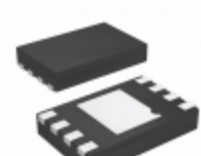
BR24G08NUX-3ATTR Rohm Semiconductor IC EEPROM 8KBIT 1MHZ 8VSON
