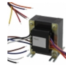
VPL28-2000 Triad Magnetics XFRMR PWR 28V 2A CHASSIS
