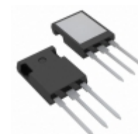
IXFR16N120P IXYS MOSFET N-CH 1200V 9A ISOPLUS247
