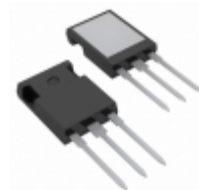
IXFR18N90P IXYS MOSFET N-CH 900V ISOPLUS247
