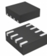
AD5620BCPZ-1500RL7 Analog Devices Inc. IC DAC 12BIT SPI/SRL 8-LFCSP
