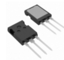
IXFX64N60P IXYS MOSFET N-CH 600V 64A PLUS247
