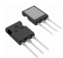
IXFX52N60Q2 IXYS MOSFET N-CH 600V 52A PLUS247
