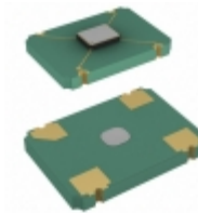
KC7050K1.84320C1GE00 AVX Corp/Kyocera Corp OSC XO 1.8432MHZ CMOS SMD
