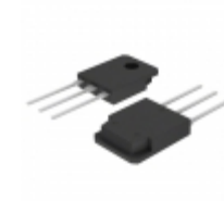
IXFH18N60X IXYS MOSFET N-CH 600V 18A TO-247
