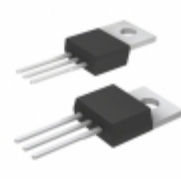
IXKP35N60C5 IXYS MOSFET N-CH 600V 35A TO-220AB
