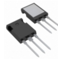
IXFR64N60P IXYS MOSFET N-CH 600V 36A ISOPLUS247
