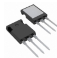
IXFR70N15 IXYS MOSFET N-CH 150V 67A ISOPLUS247
