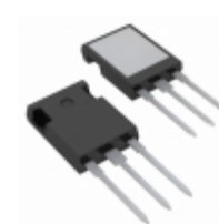
IXFR24N100 IXYS MOSFET N-CH 1KV 22A ISOPLUS247
