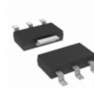
BCP 55-16 E6327 Infineon Technologies TRANS NPN 60V 1A SOT-223
