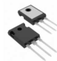
IRFPC40 Vishay Siliconix MOSFET N-CH 600V 6.8A TO-247AC
