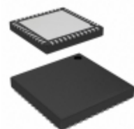
CY8C20636AN-24LTXI Cypress Semiconductor Corp IC CAPSENCE 8K FLASH 48QFN
