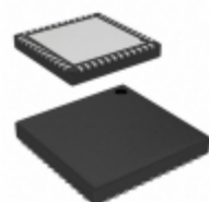
CY8C20646A-24LTXI Cypress Semiconductor Corp MCU 16K FLASH 2K SRAM 48QFN
