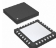
PIC18F24K20-E/ML Microchip Technology IC MCU 8BIT 16KB FLASH 28QFN
