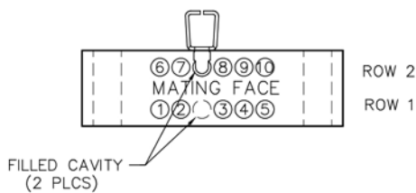
PLUG MA-211-010-161-ABCWA
