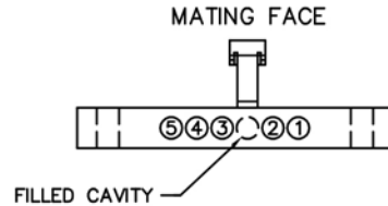
RECEPTACLE MA-121-005-261-A03WA
