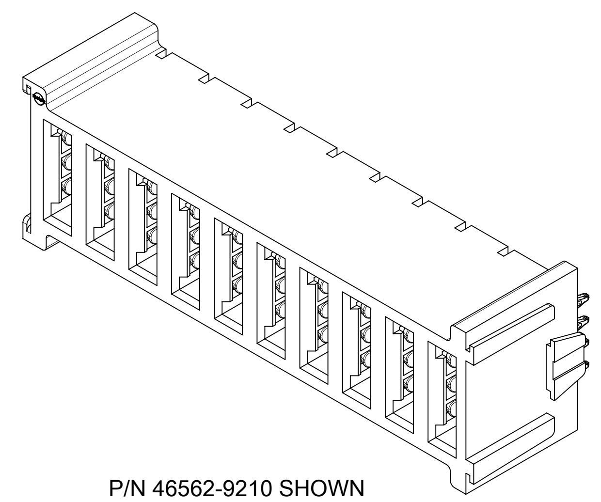
P/N 46562-9210 SHOWN
