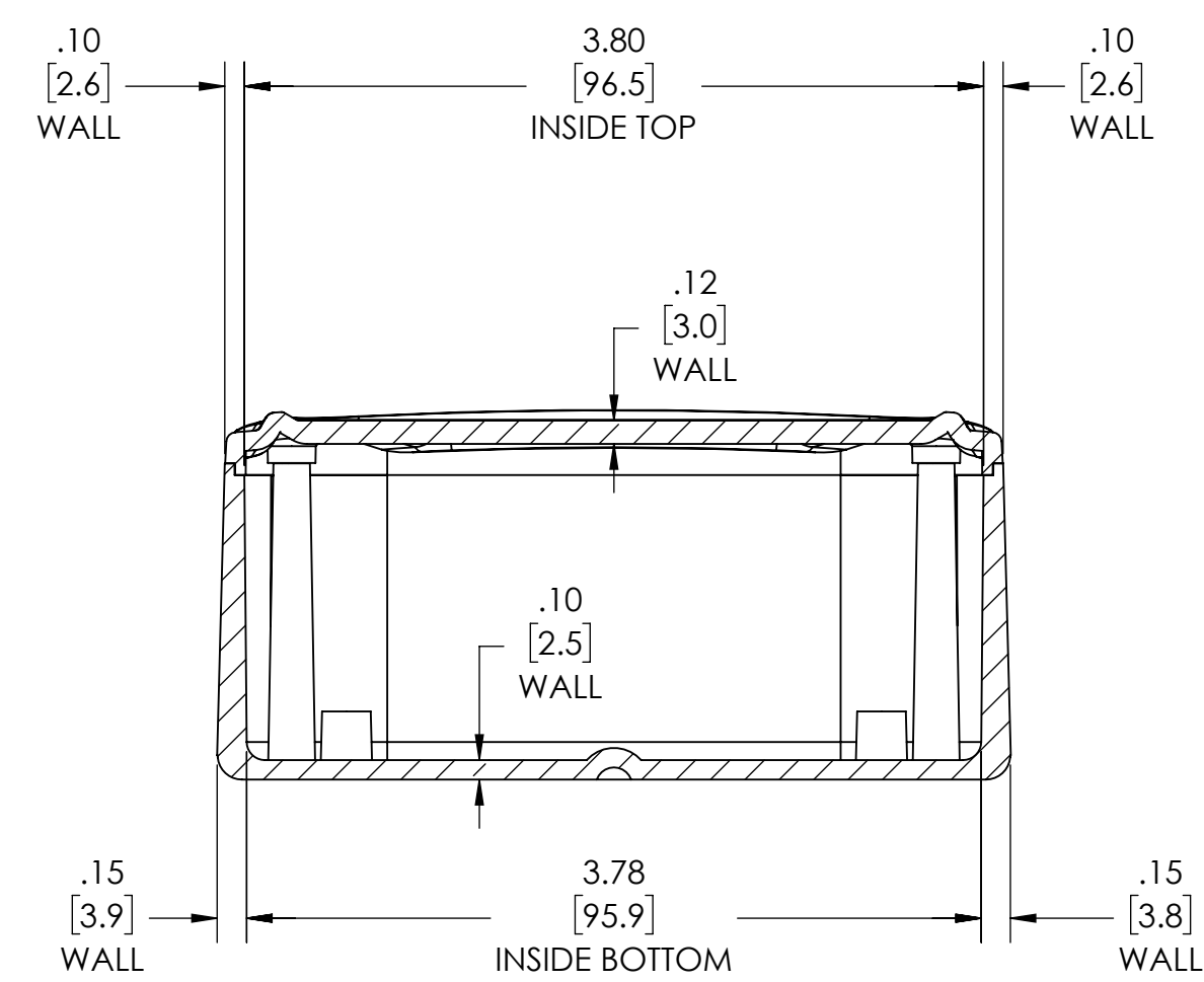
SECTION A-A
