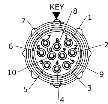
WIRING END W8882-10PG-P-5XX
