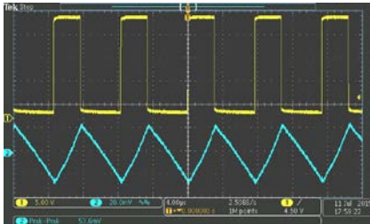
Vin=24V Vout=9V Iout=1A
