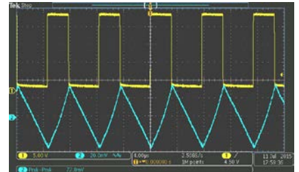
Vin=24V Vout=9V Iout=2.4A
