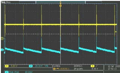
Vin=24V Vout=9V Iout=0A
