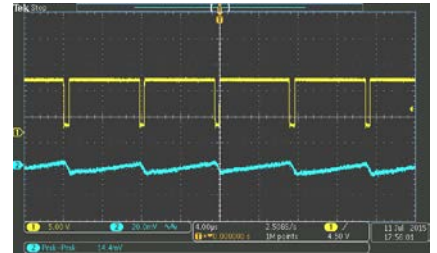
Vin=10V Vout=9V Iout=2.4A
