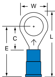
MVU14-516R/S Stud Size 5/16 Wire Range 16-14
