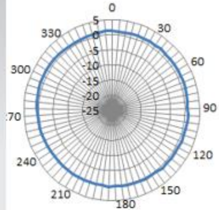
YZ-2450MHz
