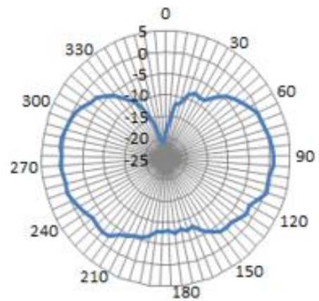
YZ-2450MHz
