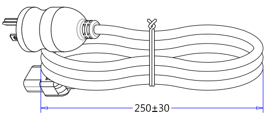
B-C3 扎線圖示 (Tied Loop Hank Detail)
