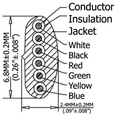
SEC: A-A
