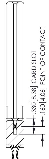
SECTION A-A
