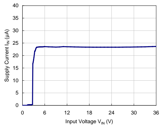
VR=3.3V
